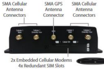
MAX HD2 Mini
