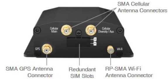
MAX Transit Mini
