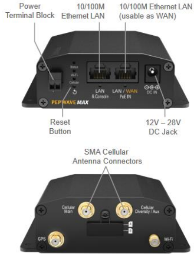
MAX BR1 Mini
